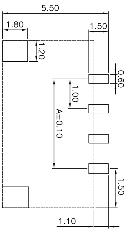
P.C.B LAYOUT
