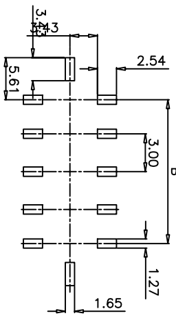
P.C.B. LAYOUT
